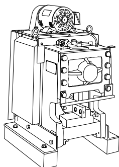
▲鉄筋切断機
