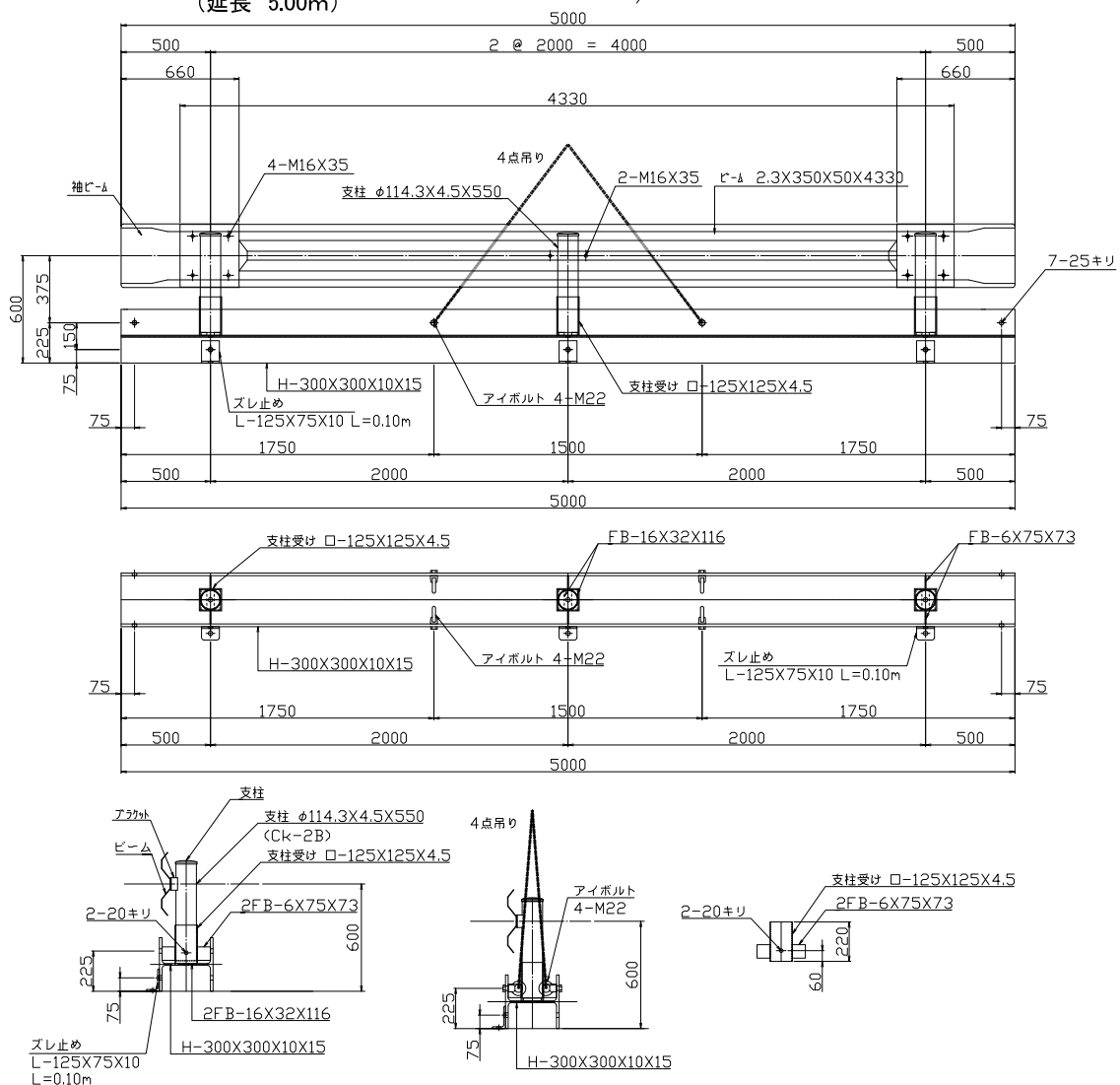
ガードレール組立図 (延長 5.00m)
